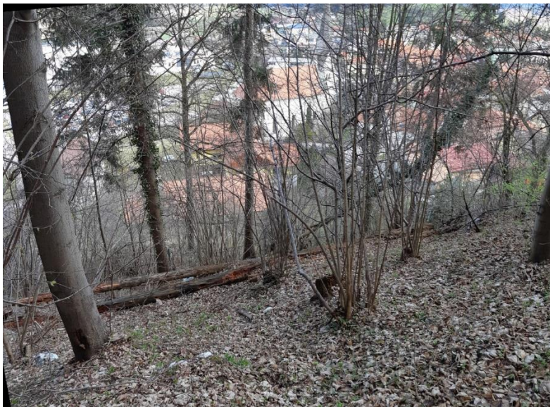
Slika 9 Območje profila P5 - podrti suhi drevesni panji za zadrževanje kotalečih skalnih blokov po terenu.
